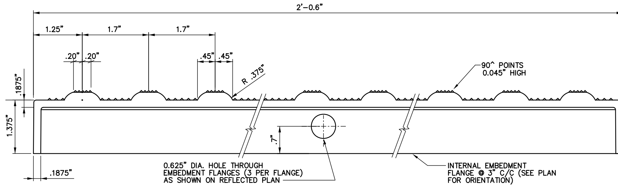
SECTION A-A
